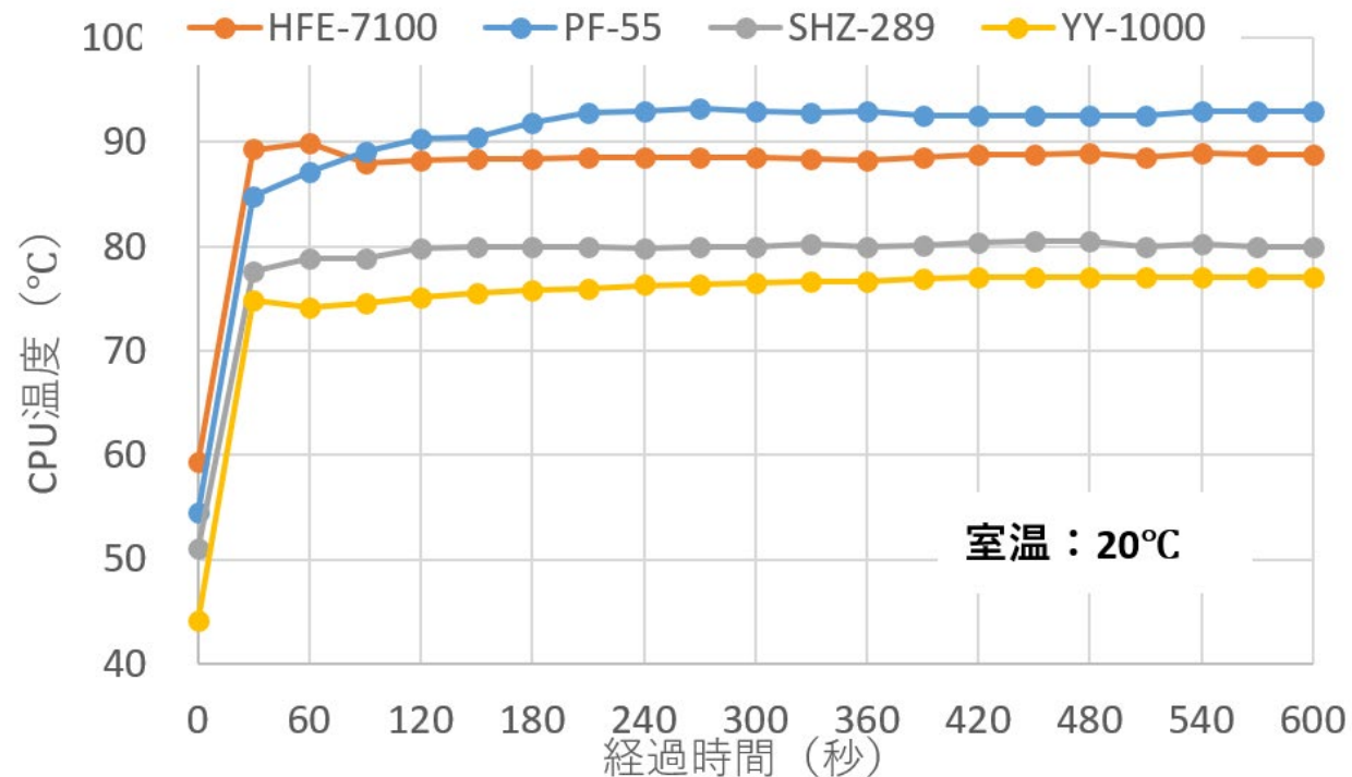
CPU温度の実測結果
